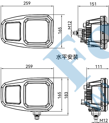
垂直安装
